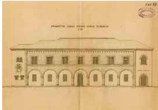
Prospetto 1913
