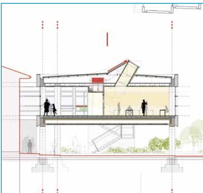
Sezione
